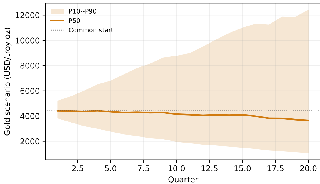
Bates-Poisson
